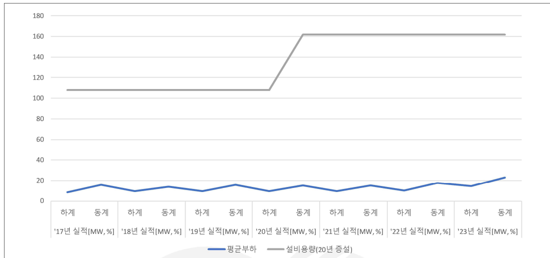
[그림 2] 154kV ☆○변전소 부하변동 추이
